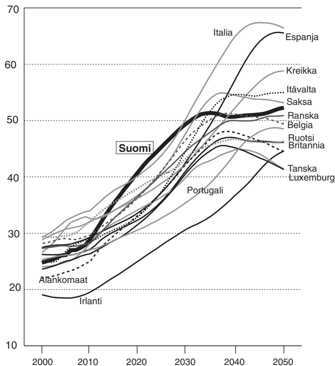
Kuvio 1. Vanhushuoltosuhte EU-maissa vuosina 2000–2050 (65 vuotta täyttäneitä sataa 20–64-vuotiaasta työikäistä kohti)
