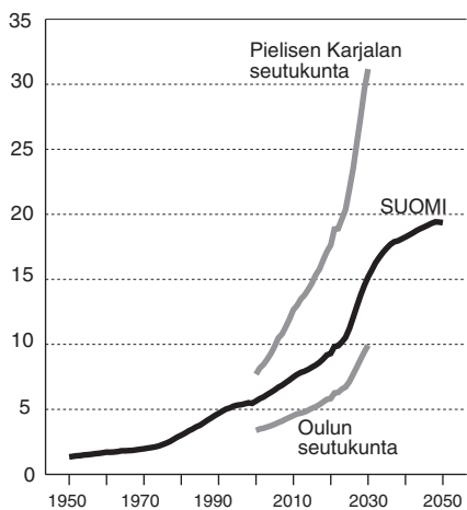
Kuvio 3. Ikähoivasuhde Suomessa 1950–2050 sekä muuttoliikelaskelman mukaan alhaisimman ja korkeimman ikähoivasuhteen seutukunnassa vuoteen 2030
