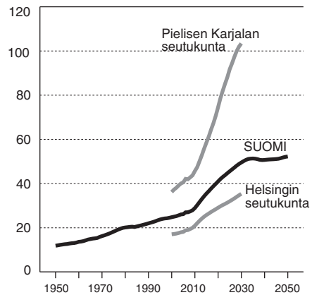
Kuvio 2. Vanhushuoltosuhte Suomessa vuosina 1950–2050 sekä Helsingin ja Pielisen Karjalan seutukunnissa vuoteen 2030
