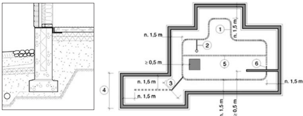
Kuva 2. Maanvaraisen laatan tiivistäminen ja radonputkiston asentaminen. Kuvat RT-ohjekortista RT 81-10791.
