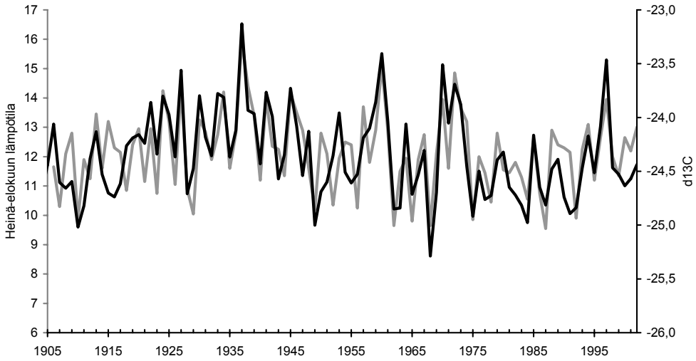
Kuva 1. Lapista, Kessin alueelta, männyistä mitattu hiilen isotooppisuhtesarja ja Inarissa mitattu lämpötila ( r=0,77 ). Musta viiva kuvaa isotooppisuhdetta ja harmaa viiva lämpötilaa.
