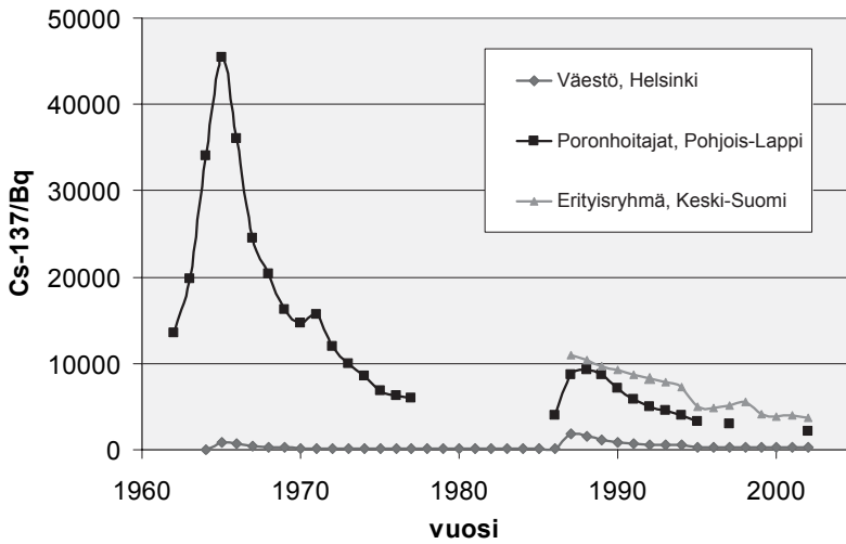
Kuva 1. 137 Cs:n määrä henkilöä kohden Helsingin väestöä edustavassa vertailuryhmässä, Pohjois-Lapin poronhoitajissa sekä paljon luonnontuotteita syövissä keski-suomalaisissa.
