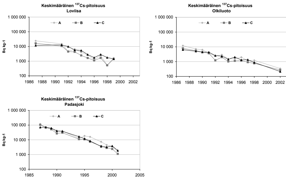
Kuva 1. Keskimääräinen ^{137}\text{Cs} -pitoisuus \text{Bq kg}^{-1} kuivapainoa kohti eri jäkälän osissa eri vuosina.
