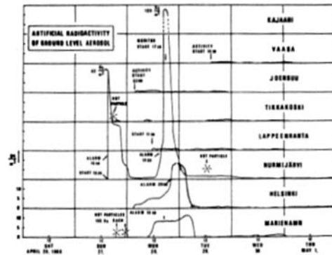
Kuva 2. Saastuneen ilman havainnot muutamalla havaintoasemalla 26.4.–1.5. 1986. Kuvan vaakaviivat kulkevat 20 Bq/m 3 välein.
