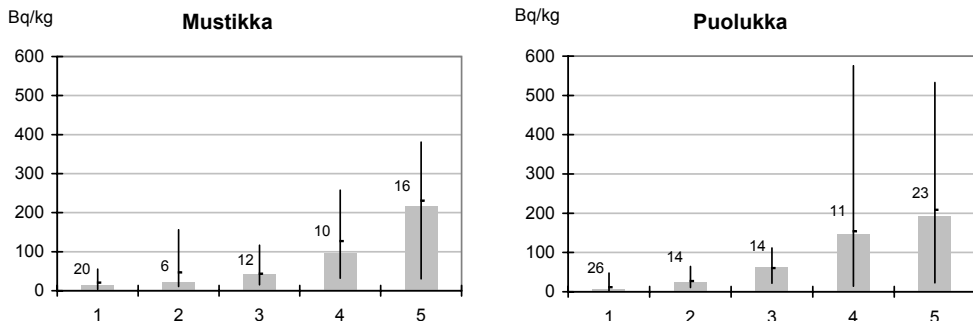
Kuva 1. ^{137}\text{Cs} :n aktiivisuuspitoisuuden keskiarvot (.), mediaanit ja vaihteluvälit tuorepaina kohti vuosina 2000–2005 mitatuissa näytteissä laskeumatasoittain. Näytteiden lukumäärä on ilmoitettu mediaanipylväiden yläpuolella.
