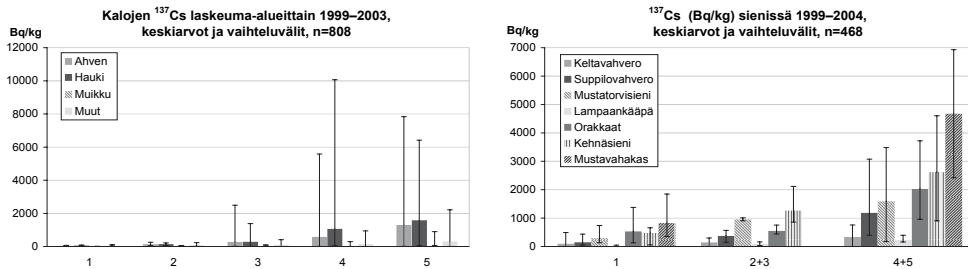
Kuva 1. Kalojen ja sienien 137 Cs-pitoisuuksia eri laskeuma-alueilta STUKissa mitatuissa näytteissä. Eniten laskeumaa tuli alueelle 5 ja vähiten alueelle 1.
