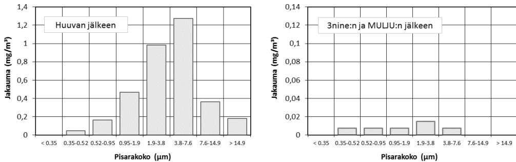
Kuva 28. Kokojakaumat huuvun jälkeen ennen erotinyhdistelmää ja yhdistelmän jälkeen.
