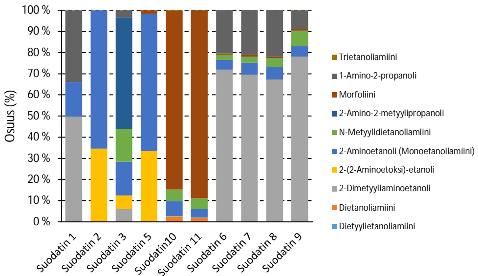
Kuva 12. Eri alkanoliamiinien osuudet suodattinyksikköjen jälkeisessä ilmassa.
